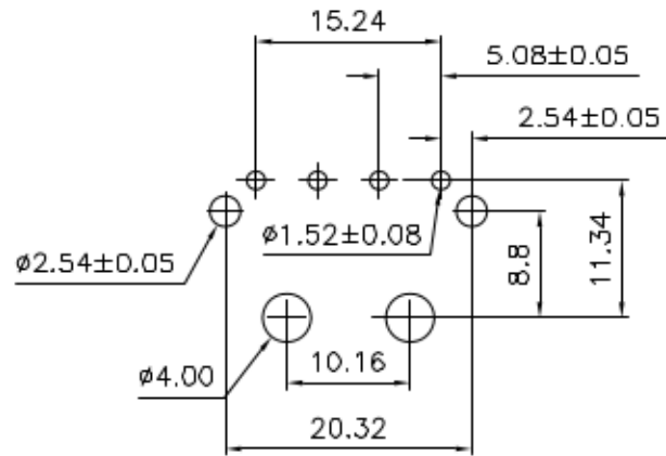
P.C.Board Layout
