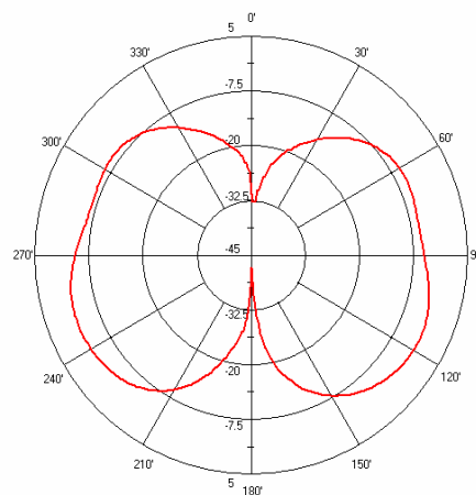
AN9520 E-Plane
