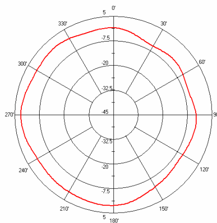
AN9520 E-Plane
